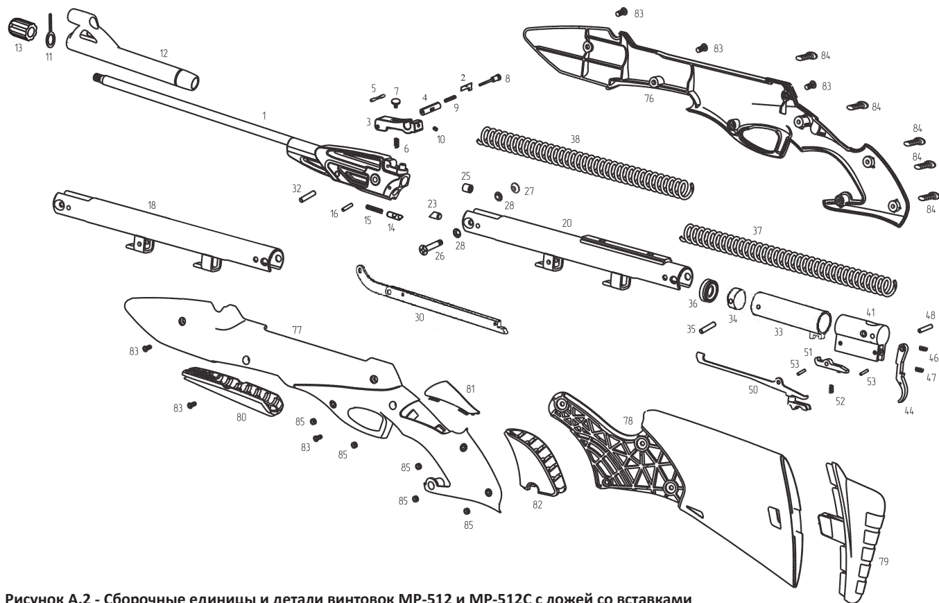
Рисунок А.2 - Сборочные единицы и детали винтовок MP-512 и MP-512C с ложей со вставками
