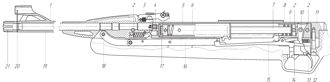
Рисунок А.6 - Схема механизмов винтовок МР-512, МР-512С с ложей со вставками
