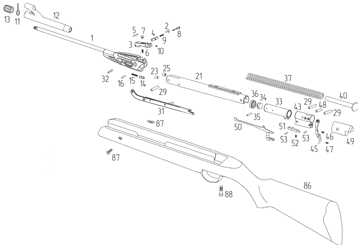
Рисунок А.3 – Сборочные единицы и детали винтовок MP-512 исполнения «Мурена»
